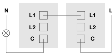
ŠVIESOS REGULIATORIUS PERJUNGKLIS
