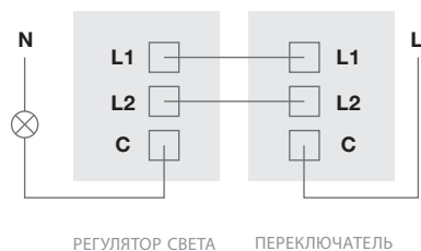
Цепь двустороннего включения
