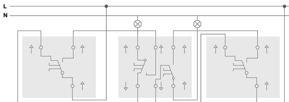
ПЕРЕКЛЮЧАТЕЛЬ 1-КЛАВИШНЫЙ
