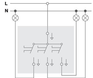
ВКЛЮЧАТЕЛЬ 3-КЛАВИШНЫЙ
